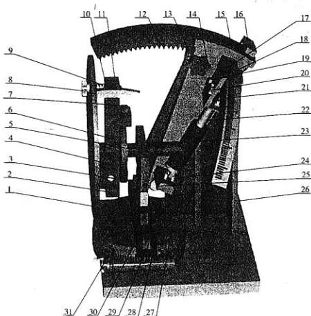
图 A.3 车轮定位角模拟机构
