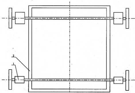
图 A.2 四轮定位仪试验台
